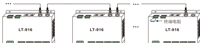
3针XLR并联连接
