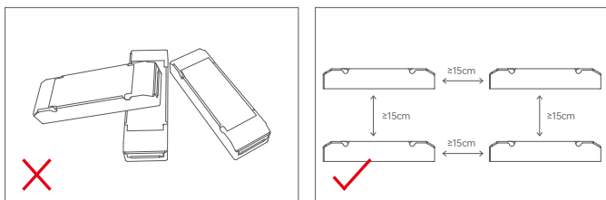
请勿将产品堆叠摆放，产品与产品间隔距离应 \geq 15\text{cm} ，避免影响产品散热和使用寿命。
