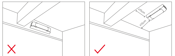
请勿将产品安装在横梁、墙角等位置，间隔距离应 \geq 15\text{cm} ，以免信号干扰影响使用。
