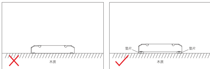
请勿将产品螺丝固定紧贴于木板，应在固定螺丝下增加 \geq 7\text{mm} 的垫片，留点空隙可以有效散热，避免影响产品散热和使用寿命。
